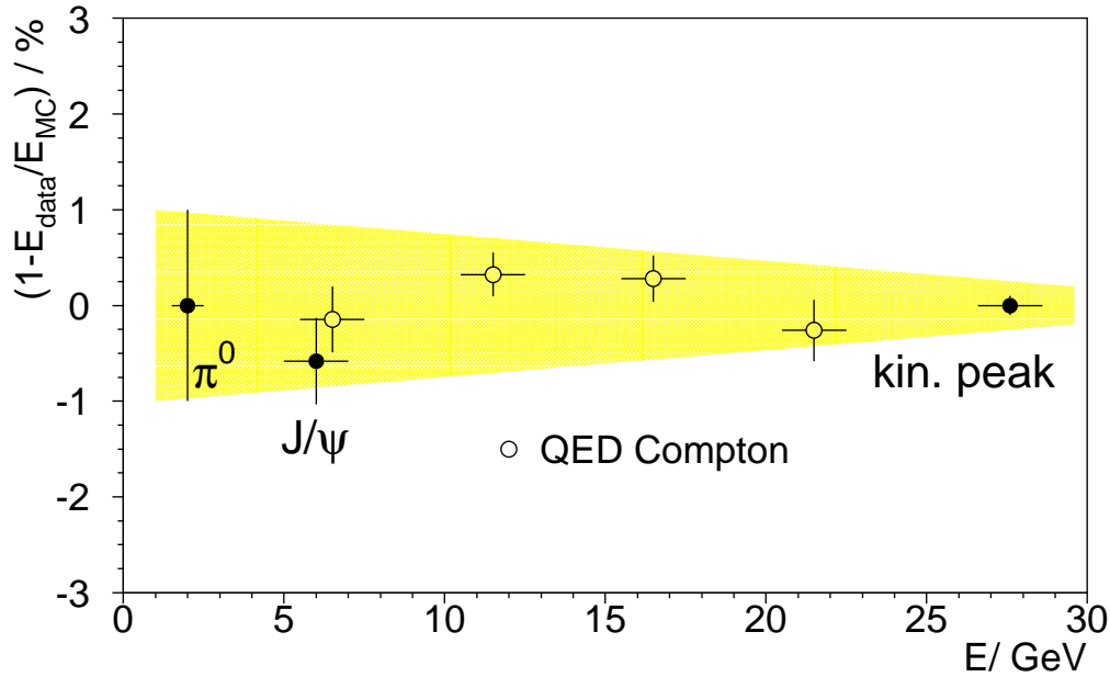
Рис. 2: Обзор определения энергетической шкалы SpaCal. Затемнённая область показывает погрешность, возникающую из-за разницы шкалы в данных и МС.
