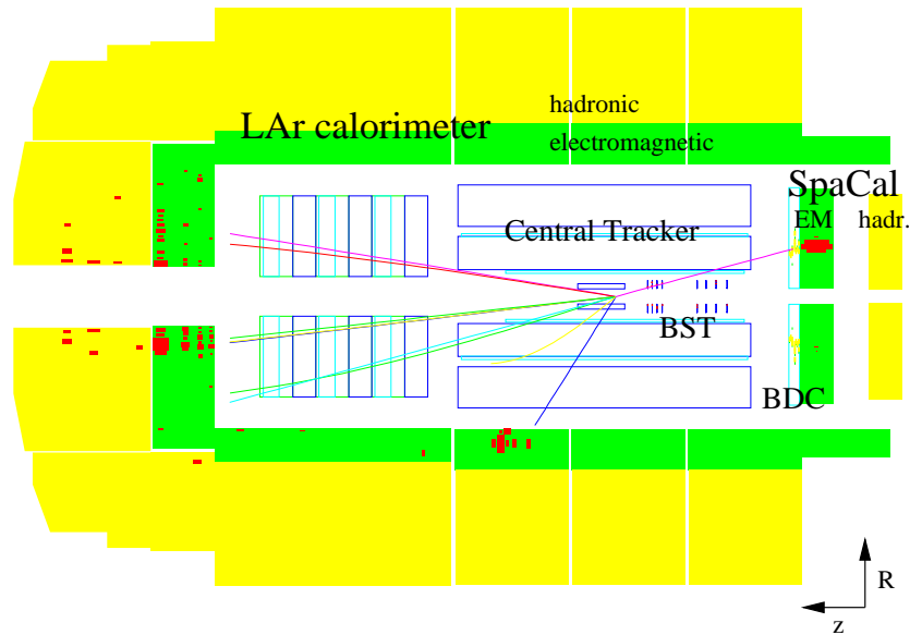
Рис. 1: Событие с малым значением Q^2 , реконструированное в детекторе H1. Электрон рассеивается в заднюю область. Его траектория реконструирована в Backward Silicon Tracker (BST) и в Backward Drift Chamber (BDC). Энергия электрона определена в калориметре SpaCal. Конечное адронное состояние зарегистрировано в центральном и переднем трековых детекторах, а так же в калориметре LAr.
