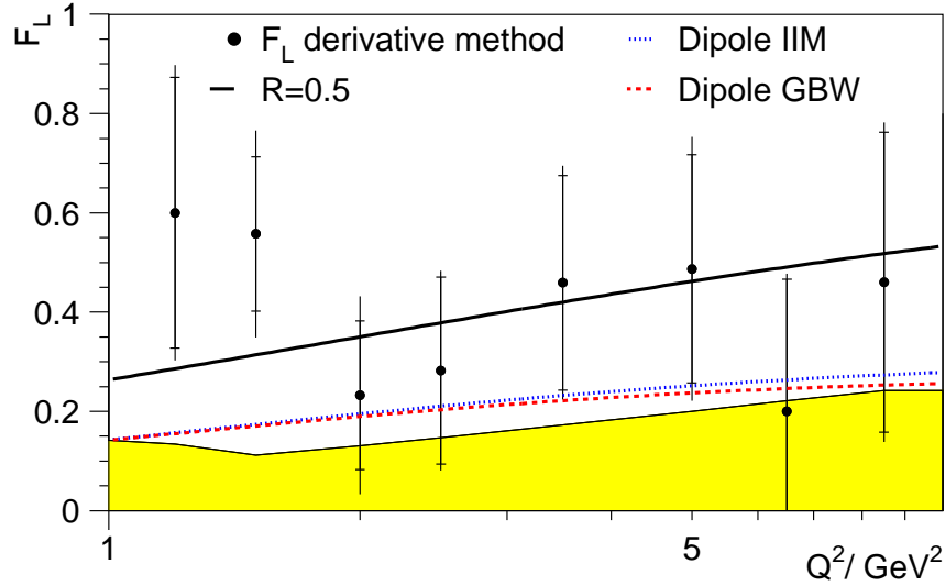
Рис. 5: Структурная функция F_L , полученная с использованием деривативного метода. Линии соответствуют R = 0.5 (чёрная), дипольной GBW (штриховая) и дипольной ИМ (пунктирная) моделям. Внутренние пределы ошибок показывают статистические погрешности, внешние – статистические и систематические погрешности, которые просуммированы квадратично. Жёлтая область соответствует неопределённости модели.
